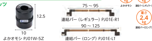
よかオモシ PJ01W-5Z
