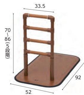
重さ 17 kg サイドタイプ PJ01-AL
